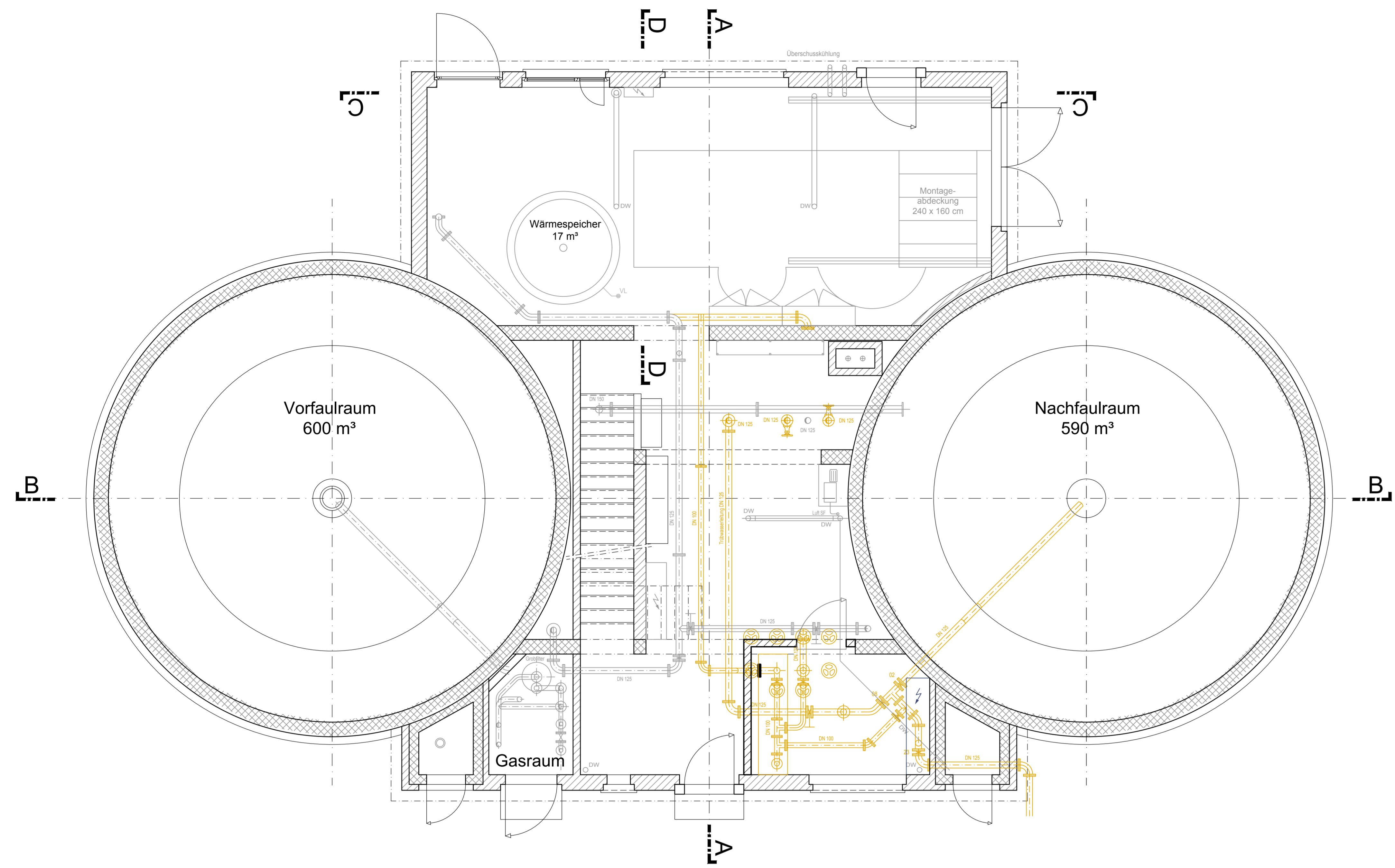
Grundriss EG
