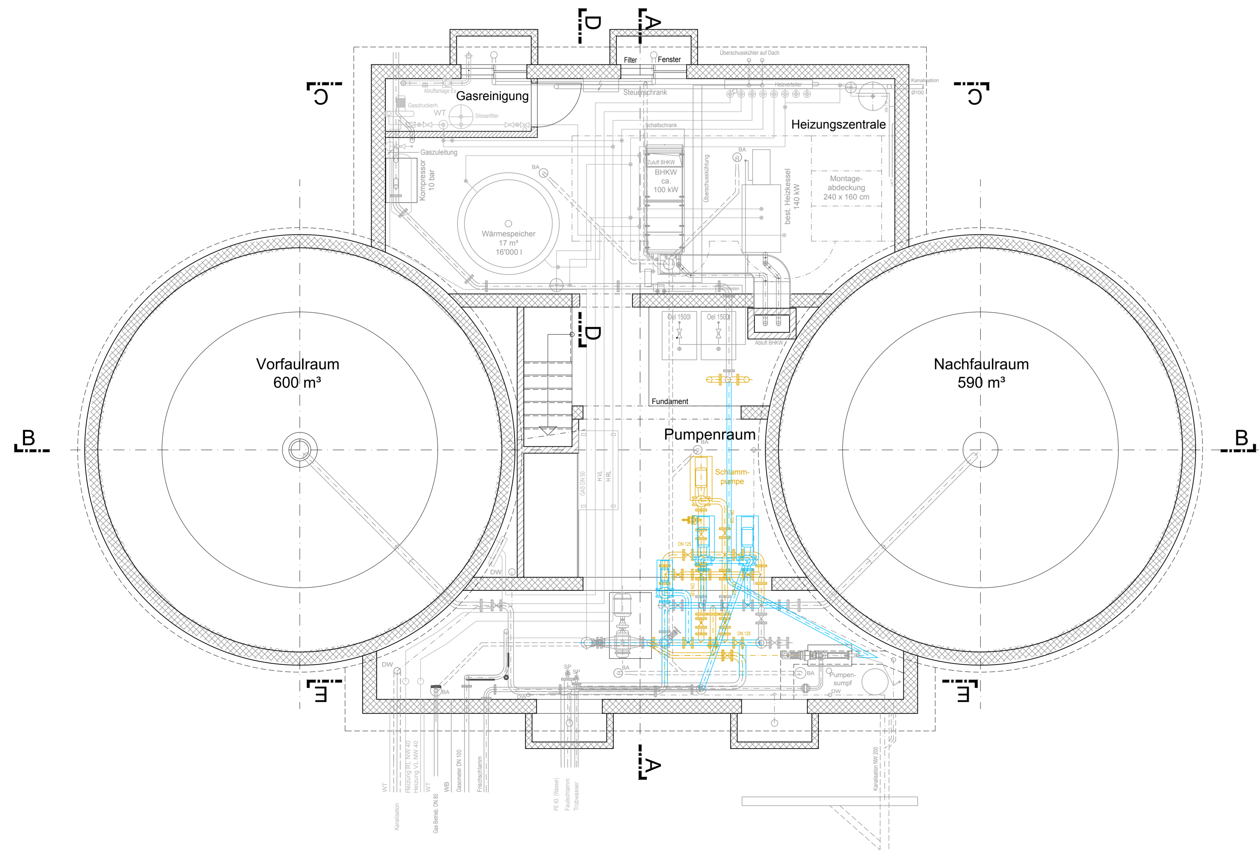
Grundriss UG
