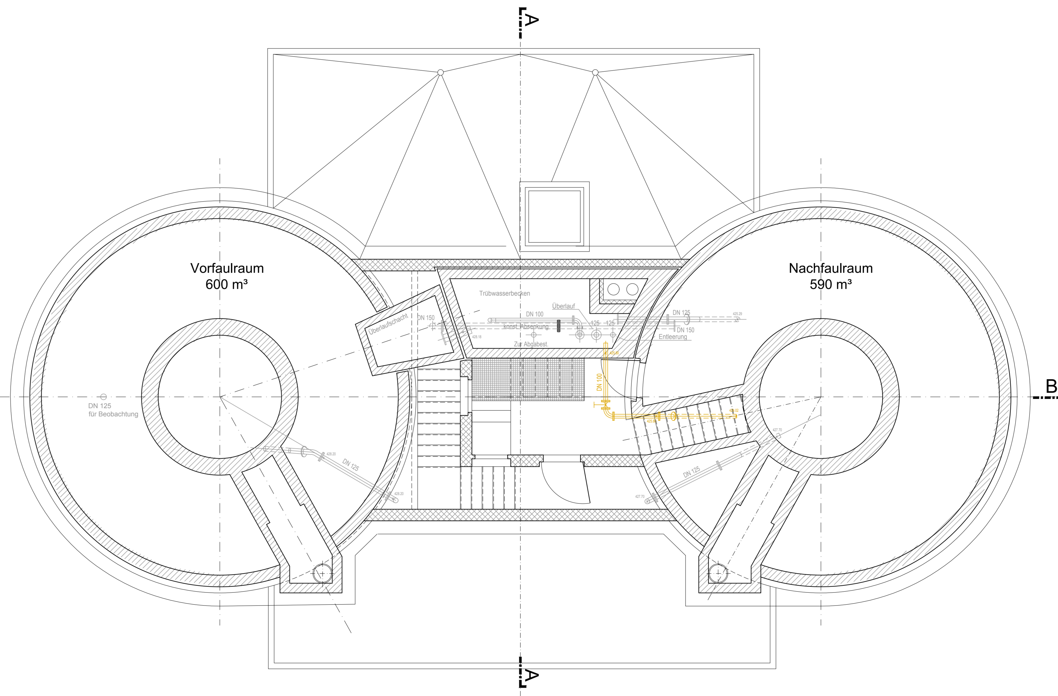
Grundriss OG
