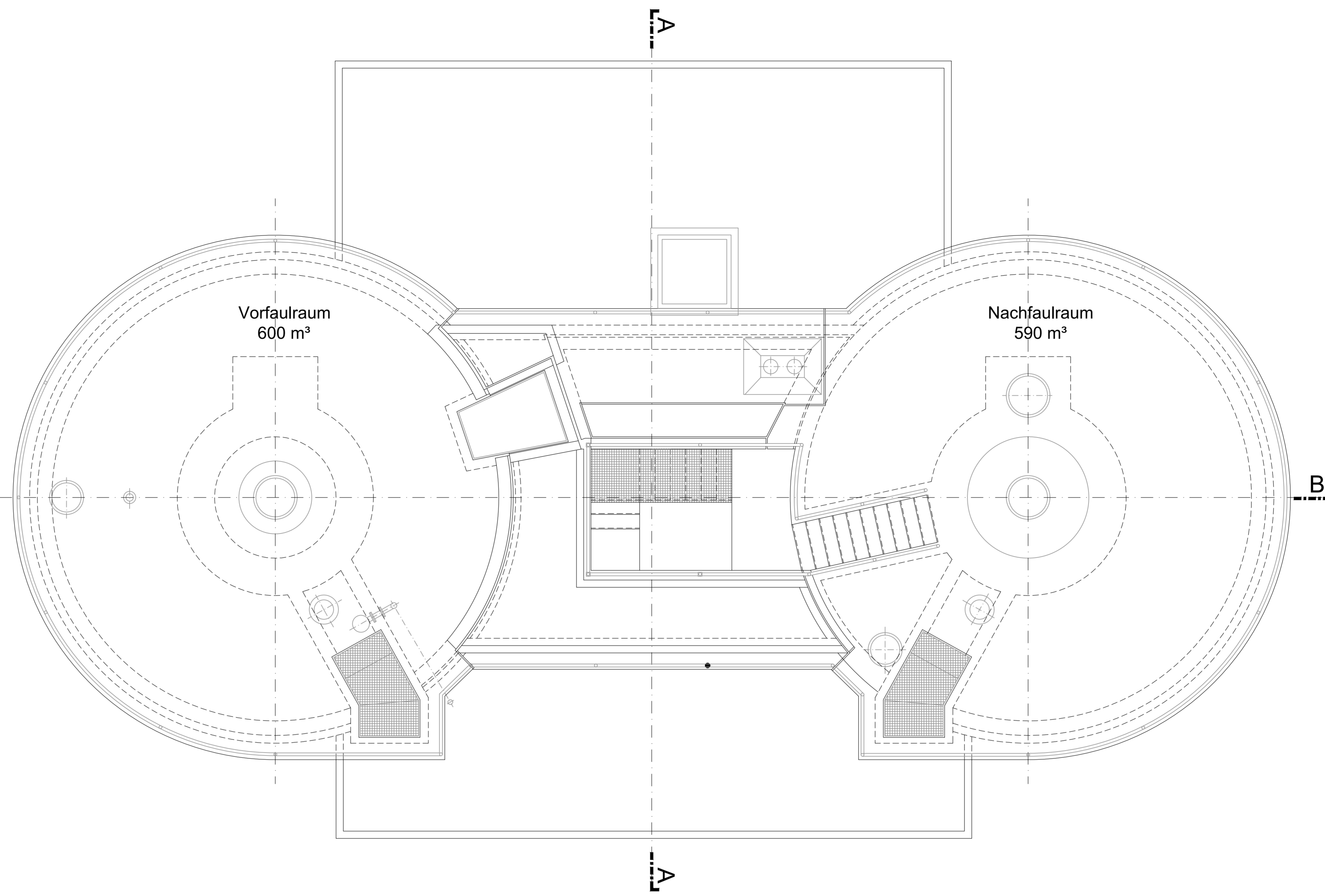
Grundriss DG
